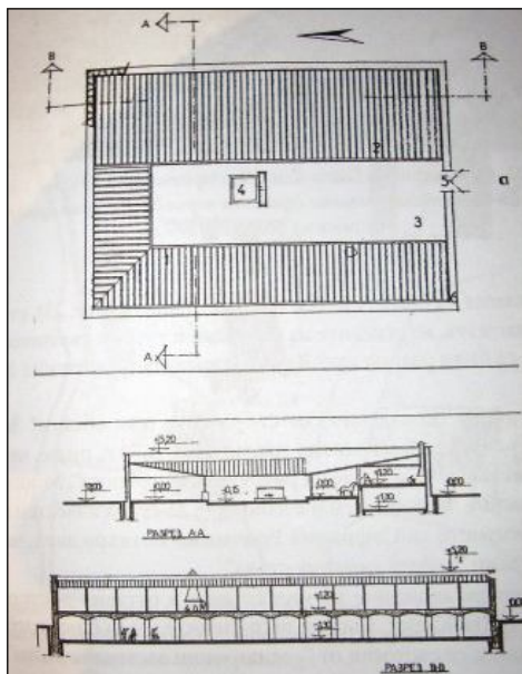
Фиг. 7. Схема на хана на Михал бей. Направена е по сведения на акад. Ю. Трифонов, пътешественици и столетници
